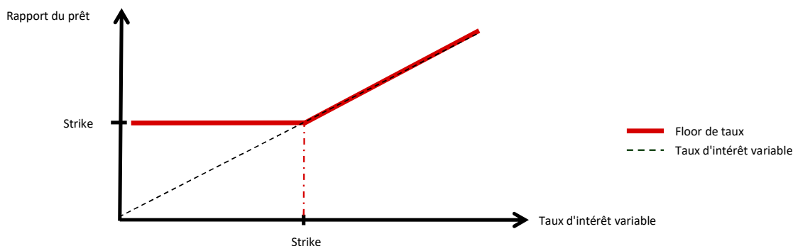
Profil d'endettement de l'acheteur du Floor de Taux (hors coût de la prime)
